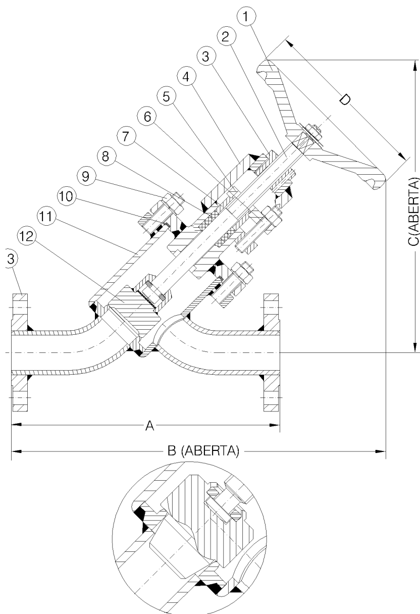
Detalhe mod. VOR-F (regulável)
