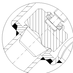
Detalhe Mod. "VOR-S" (regulável)
